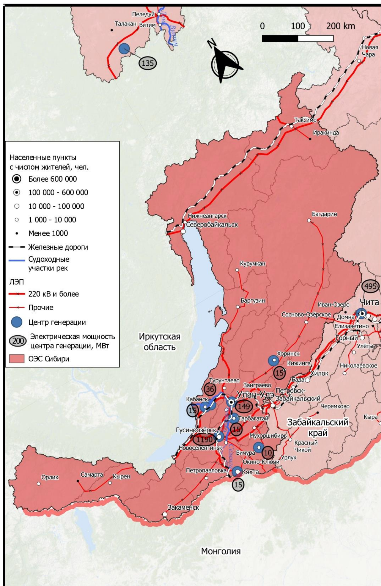
Рис. 3. Энергосистема Республики Бурятия
